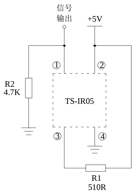
DC 5V 典型应用电路
